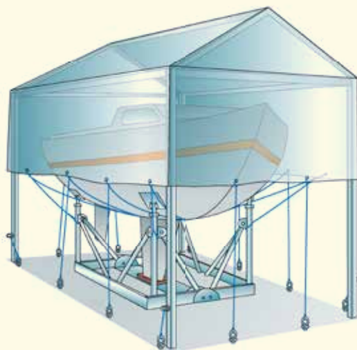
Båt med väl förankrat presenningshus.
